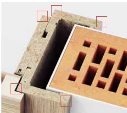
SM podboj z ostrimi robovi
