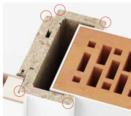
SMS podboj z vsemi zaokroženimi robovi
