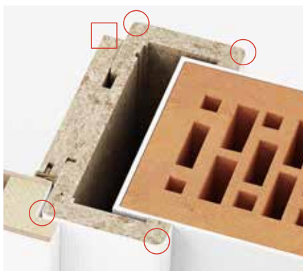
SMO podboj z zaokroženimi robovi oblog
