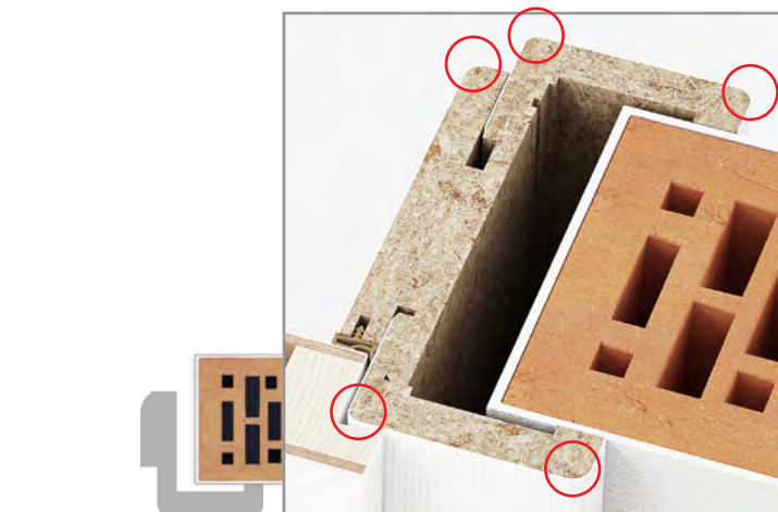
SMS podboj z vsemi zaokroženimi robovi
