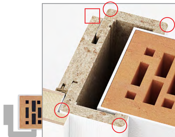
SMO podboj z zaokroženimi robovi oblog
