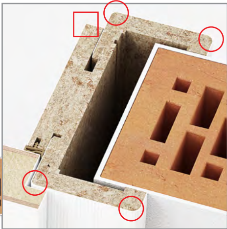
SMO podboj z zaokroženimi robovi oblog
